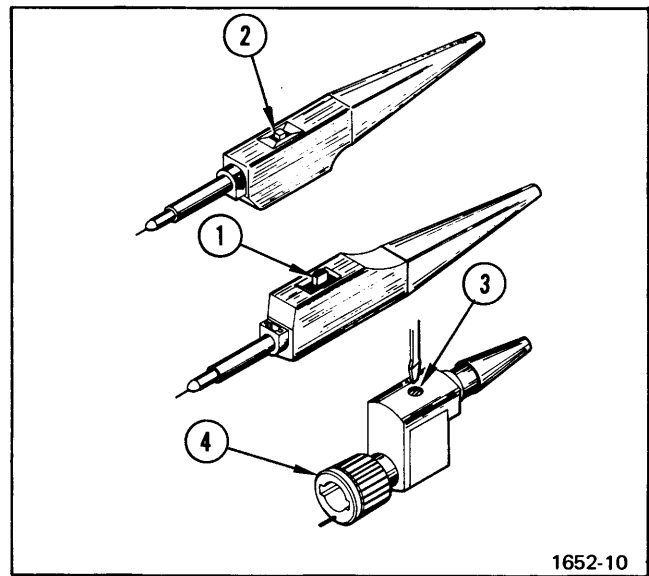
Fig. 2-7. P6062A Probe.
