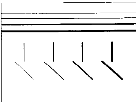
Fig. 12 100 Hz TEST, 625 / 525 Zeilen, Bildformat 4:3
