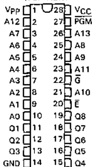
PIN NOMENCLATURE
