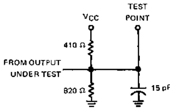
FIGURE 1A - PE OUTPUT LOAD CIRCUIT
