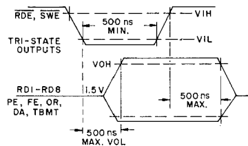
Fig.21 RDE, SWE
