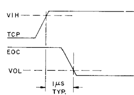
Fig.19 EOC TURN-OFF
