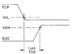
Fig.17 EOC TURN-ON
