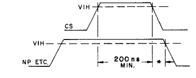
Fig.37c
