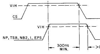
Fig.15a CS
