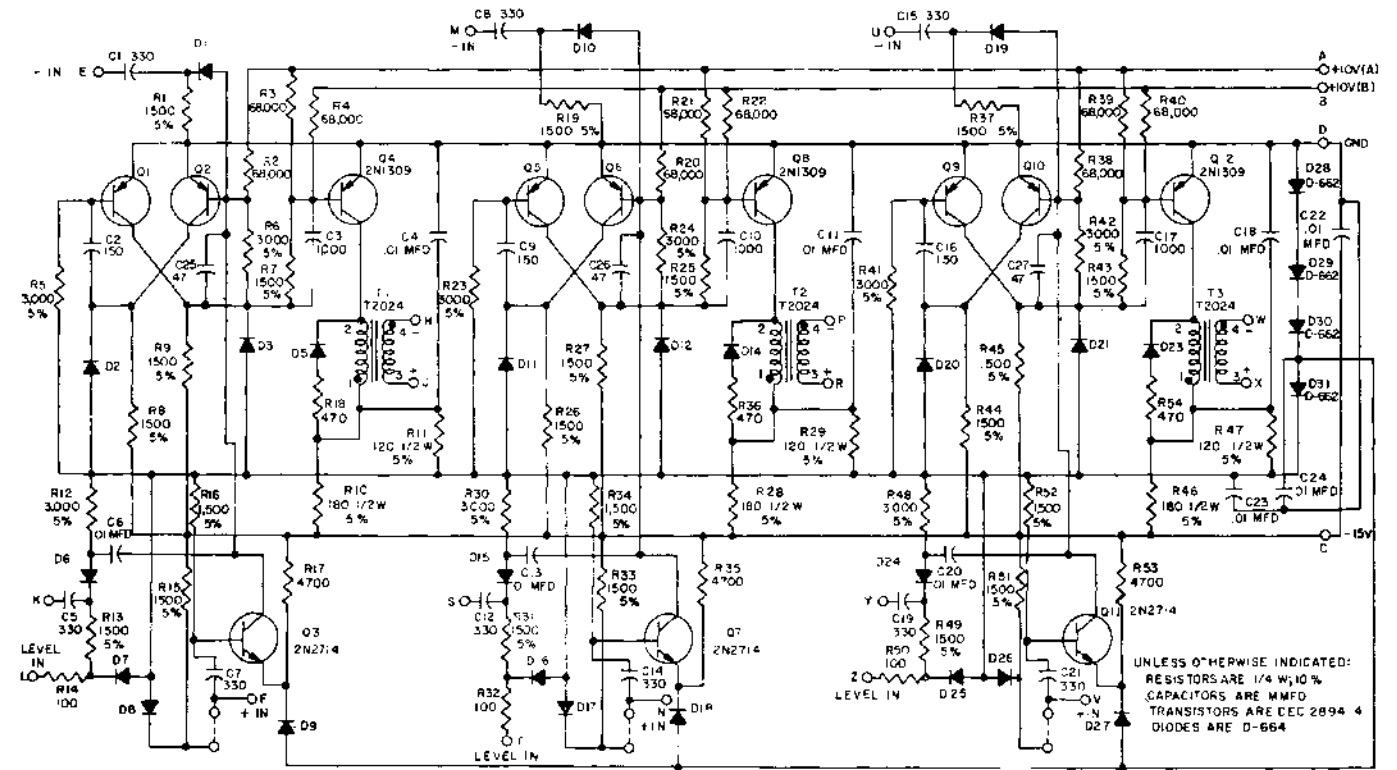
Pulse Amplifier RS-4606
