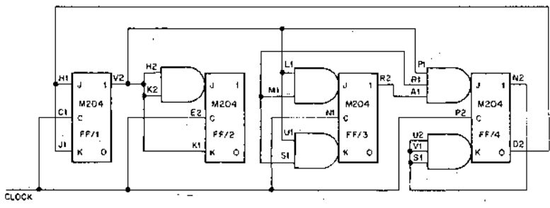
MODULUS 9
