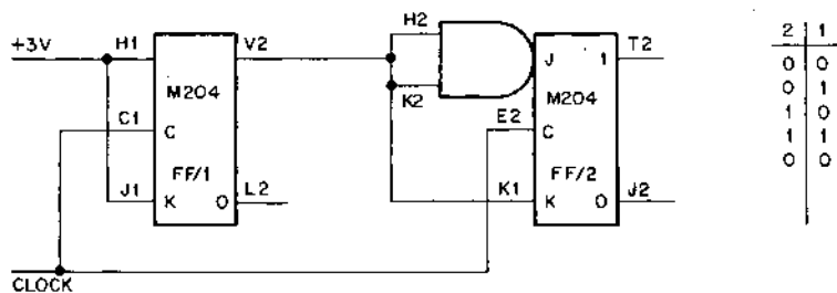
MODULUS 4
