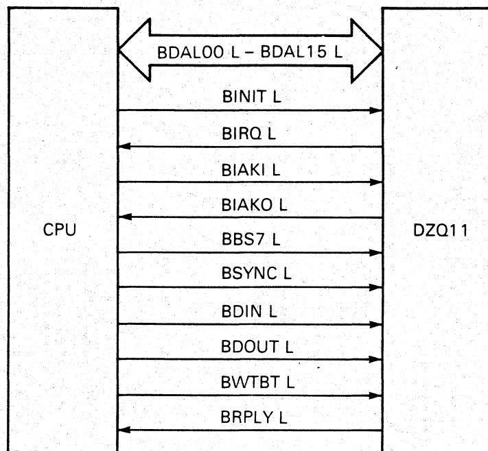
Figure 5-3 DZQ11/Q-bus Interface
