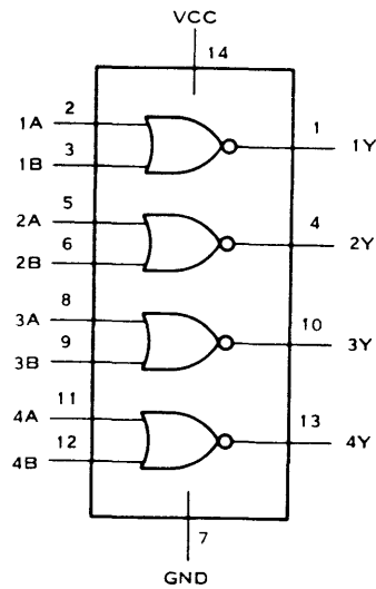
SN7402
