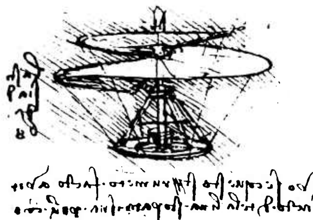
Leonardo Da Vinci: Airscrew, c.1488 (Wallace 4 )
