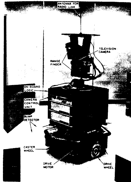
Figure 2-1: Shakey - Moravec 81b
