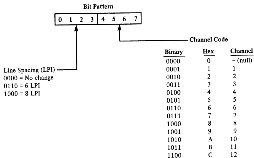
Figure 66. 4248 FCB Module Data Byte
