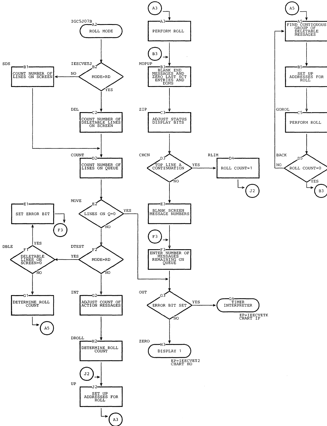
Chart HR. DIOCS Roll Mode Routine
