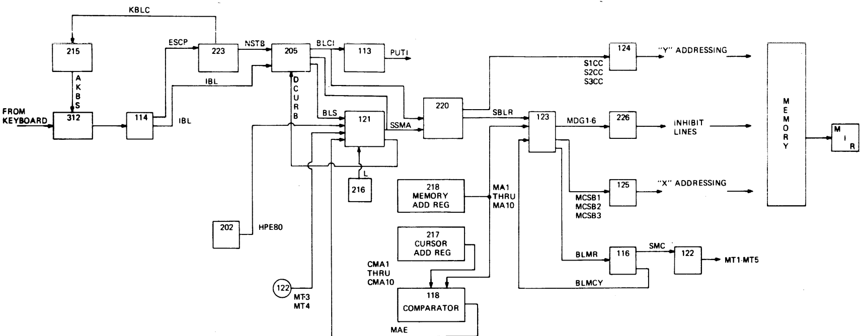
Fig. II-48 BACKLINE
