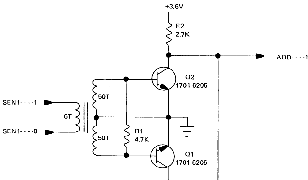
Fig. III-29 TRANSLATOR SENSE AMP.
