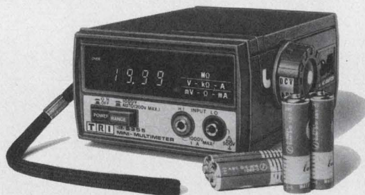
Model: 6355 Mini-multimeter
