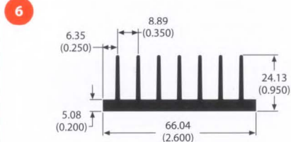
67835 1.0 lb/ft 4.45 °C/W/3in Per.=15.72
