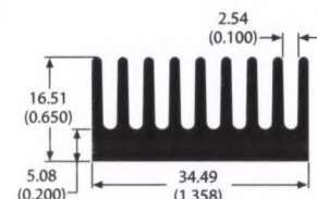
80250 0.6 lb/ft 6.61 °C/W/3in Per.=10.57
