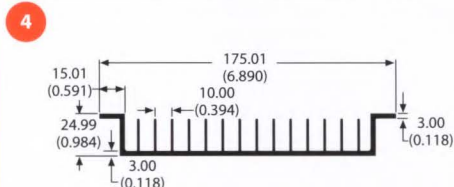
81520 3.2 lb/ft 2.55 °C/W/3in Per.=27.47
