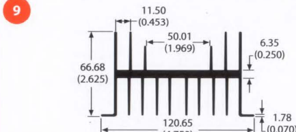
67075 2.8 lb/ft 1.56 °C/W/3in Per.=44.72
