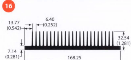
71395 4.3 lb/ft 1.21 °C/W/3in Per.=57.72
