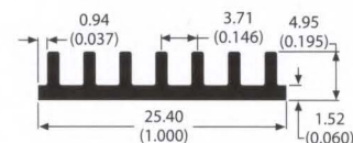
81405 0.1 lb/ft 17.98 °C/W/3in Per.=3.89
