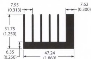
76550 1.3 lb/ft 4.36 °C/W/3in Per.=16.03
