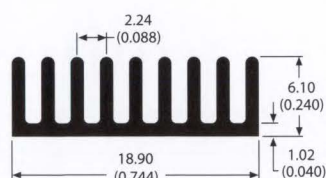
61995 0.1lb/ft 14.24 °C/W/3in Per.=4.91
