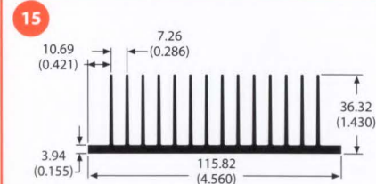
70195 2.1 lb/ft 1.58 °C/W/3in Per.=44.19
