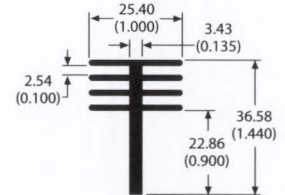
68255 0.5 lb/ft 7.13 °C/W/3in Per.=9.80
