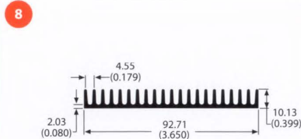
62650 0.9 lb/ft 3.66 °C/W/3in Per.=19.08
