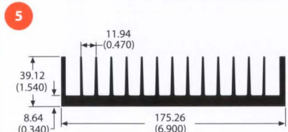
79190 1.9 lb/ft 1.85 °C/W/3in Per.=37.89
