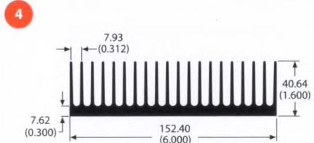
72385 4.8 lb/ft 1.13 °C/W/3in Per.=61.82
