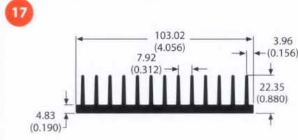
63115 1.7 lb/ft 2.76 °C/W/3in Per.=25.37
