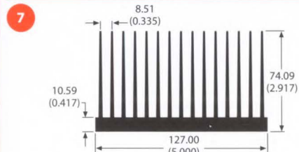
82525 6.3 lb/ft 0.83 °C/W/3in Per.=84.44
