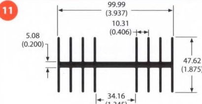
60500 2.1 lb/ft 2.05 °C/W/3in Per.=34.16
