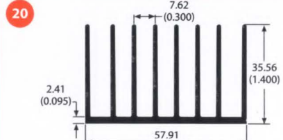
81915 1.0 lb/ft 2.77 °C/W/3in Per.=25.21
