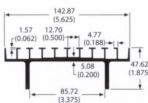
60925 2.1 lb/ft 2.31 °C/W/3in Per.=30.23
