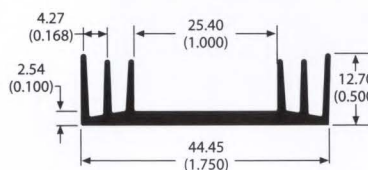
80505 0.4 lb/ft 8.74 °C/W/3in Per.=8.00
