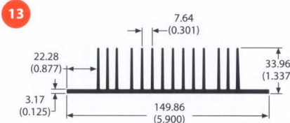
75700 2.3 lb/ft 1.56 °C/W/3in Per.=44.89
