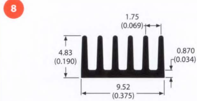
80455 0.1 lb/ft 27.50 °C/W/3in Per.=2.54
