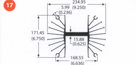
61015 9.6 lb/ft 0.60 °C/W/3in Per.=117.39
