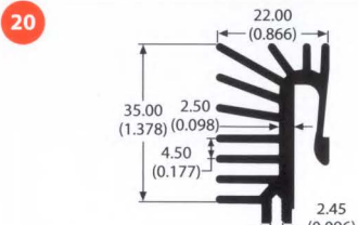
78240 0.4 lb/ft 5.51 °C/W/3in Per.=12.69
