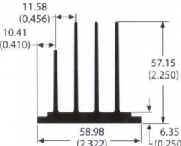
67360 1.4 lb/ft 3.59 °C/W/3in Per.=19.47
