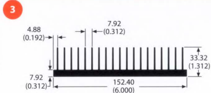
68995 3.6 lb/ft 1.41 °C/W/3in Per.=49.68
