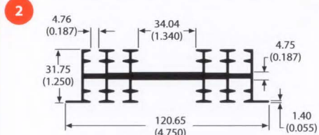
60245 1.7 lb/ft 2.11 °C/W/3in Per.=33.14
