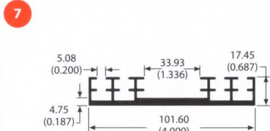
60665 1.2 lb/ft 3.48 °C/W/3in Per.=20.11
