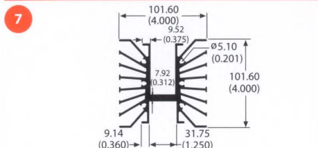
60255 4.6 lb/ft 1.09 °C/W/3in Per.=64.06
