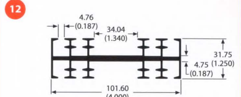
60645 1.6 lb/ft 2.28 °C/W/3in Per.=30.67
