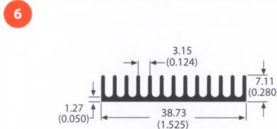
79925 0.7 lb/ft 5.98 °C/W/3in Per.=11.69
