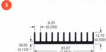
65035 0.7 lb/ft 5.16 °C/W/3in Per.=13.55
