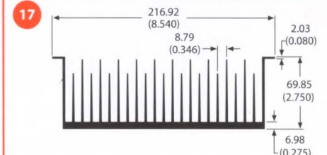
76370 7.0 lb/ft 0.61 °C/W/3in Per.=114.04
