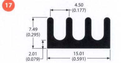
81395 0.1 lb/ft 24.85 °C/W/3in Per.=2.81
