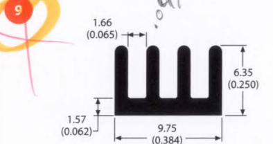
82290 0.1 lb/ft 30.53 °C/W/3in Per.=2.29
