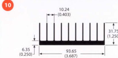
60485 1.8 lb/ft 2.56 °C/W/3in Per.=27.36
