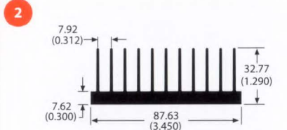
67590 1.5 lb/ft 1.58 °C/W/3in Per.=44.36
