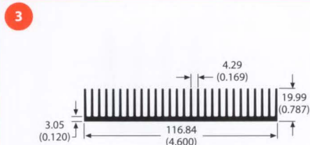
74535 1.8 lb/ft 1.55 °C/W/3in Per.=45.22
