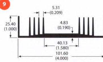
61030 1.2 lb/ft 2.90 °C/W/3in Per.=24.10
