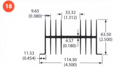
60835 2.2 lb/ft 1.54 °C/W/3in Per.=45.37
