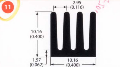
70920 0.1 lb/ft 20.43 °C/W/3in Per.=3.42
