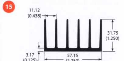
61460 0.9 lb/ft 3.96 °C/W/3in Per.=17.67
