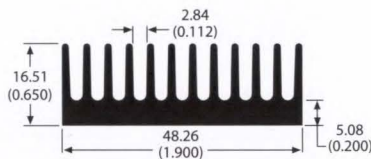
80060 0.8 lb/ft 4.96 °C/W/3in Per.=14.10
