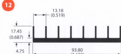
82055 1.1 lb/ft 4.51 °C/W/3in Per.=15.50
