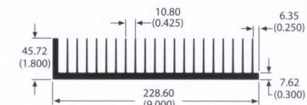
65440 6.0 lb/ft 0.87 °C/W/3in Per.=80.10
