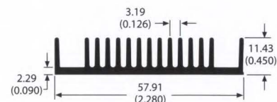
81920 0.6 lb/ft 4.75 °C/W/3in Per.=14.73
