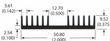
61420 0.4 lb/ft 6.83 °C/W/3in Per.=10.24
