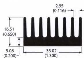
81130 0.6 lb/ft 7.31 °C/W/3in Per.=9.57
