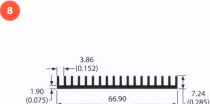
68145 0.4 lb/ft 5.65 °C/W/3in Per.=12.37
