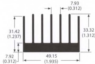
62815 1.2 lb/ft 3.91 °C/W/3in Per.=17.88
