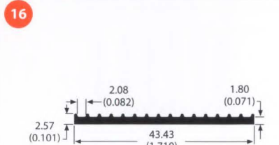
80190 0.2 lb/ft 16.96 °C/W/3in Per.=4.12
