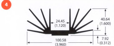
60070 0.4 lb/ft 6.96 °C/W/3in Per.=10.05
