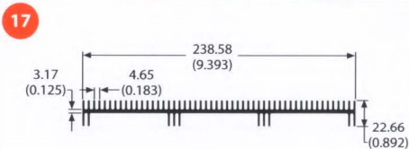
62160 3.1 lb/ft 1.01 °C/W/3in Per.=69.24
