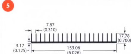
72385 4.8 lb/ft 1.13 °C/W/3in Per.=61.82
