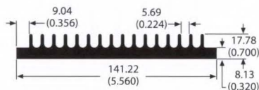
65325 2.8 lb/ft 3.21 °C/W/3in Per.=21.81
