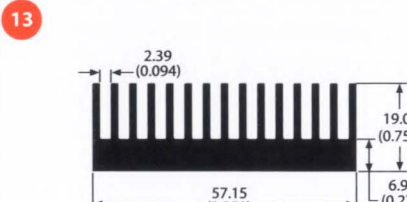
75625 1.2 lb/ft 3.67 °C/W/3in Per.=19.05
