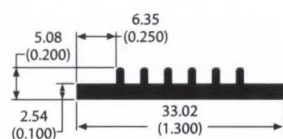
74200 0.2 lb/ft 17.95 °C/W/3in Per.=3.90
