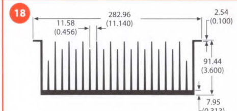
76375 10.6 lb/ft 0.45 °C/W/3in Per.=153.80
