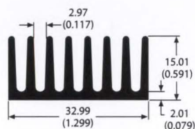
80720 0.5 lb/ft 6.81 °C/W/3in Per.=10.27
