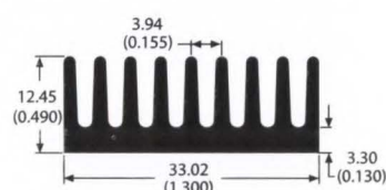
79200 0.5 lb/ft 8.05 °C/W/3in Per.=8.69
