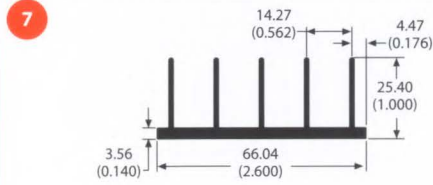
67835 1.0 lb/ft 4.45 °C/W/3in Per.=15.72
