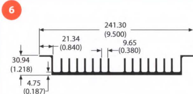
70455 3.1 lb/ft 2.24 °C/W/3in Per.=31.22
