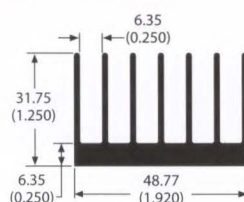
62745 1.1 lb/ft 3.88 °C/W/3in Per.=18.00
