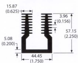
78610 2.0 lb/ft 2.91 °C/W/3in Per.=24.06
