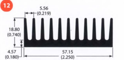
79820 1.0 lb/ft 4.35 °C/W/3in Per.=16.06
