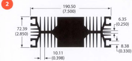
63880 14.9 lb/ft 0.78 °C/W/3in Per.=89.61
