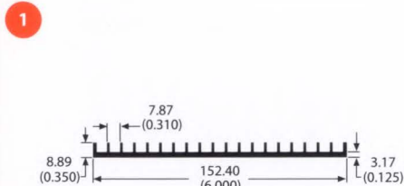
62995 1.2 lb/ft 3.34 °C/W/3in Per.=20.92
