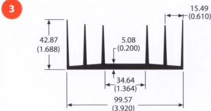
61050 1.5 lb/ft 2.87 °C/W/3in Per.=24.37
