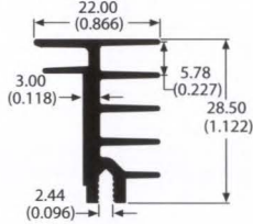
78265 0.3 lb/ft 8.72 °C/W/3in Per.=8.02
