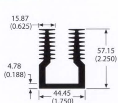
60180 1.9 lb/ft 2.94 °C/W/3in Per.=23.82
