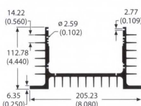
65130 6.2 lb/ft 1.06 °C/W/3in Per.=66.19
