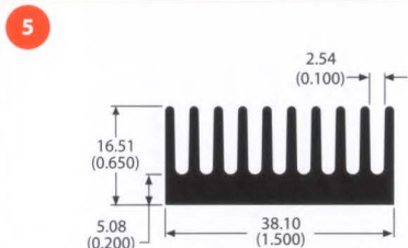
79925 0.7 lb/ft 5.98 °C/W/3in Per.=11.69
