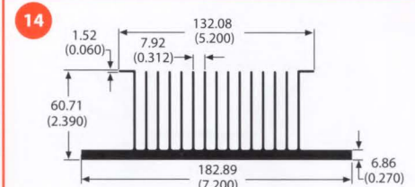
class A 62625 4.5 lb/ft 0.89 °C/W/3in Per.=78.20
