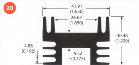
60525 1.1 lb/ft 5.85 °C/W/3in Per.=11.95
