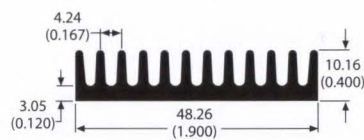
81295 0.6 lb/ft 7.12 °C/W/3in Per.=9.82
