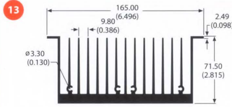
75560 6.3 lb/ft 0.83 °C/W/3in Per.=84.51
