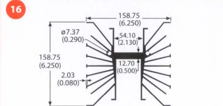
79240 7.6 lb/ft 0.65 °C/W/3in Per.=108.30
