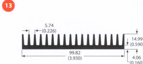
79980 1.5 lb/ft 3.18 °C/W/3in Per.=21.99
