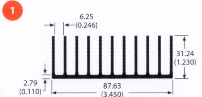
67590 1.5 lb/ft 1.58 °C/W/3in Per.=44.36
