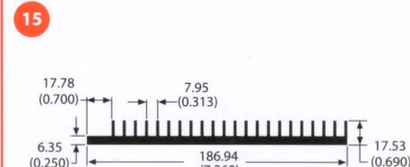
66880 4.1 lb/ft 1.18 °C/W/3in Per.=59.05
