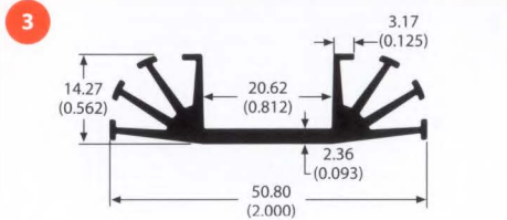
60070 0.4 lb/ft 6.96 °C/W/3in Per.=10.05
