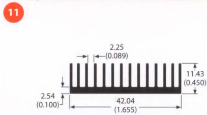
82495 0.4 lb/ft 5.35 °C/W/3in Per.=13.07
