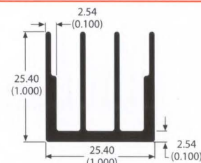
80765 0.4 lb/ft 7.61 °C/W/3in Per.=9.19
