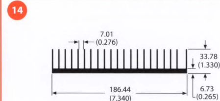
66880 4.1 lb/ft 1.18 °C/W/3in Per.=59.05
