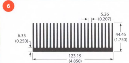
82030 5.2 lb/ft 0.87 °C/W/3in Per.=80.42
