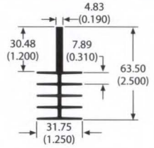
61150 1.2 lb/ft 4.35 °C/W/3in Per.=16.07
