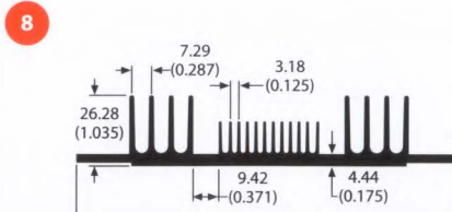
81760 2.0 lb/ft 2.02 °C/W/3in Per.=34.55
