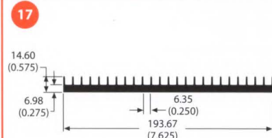
63350 3.1 lb/ft 2.38 °C/W/3in Per.=29.32
