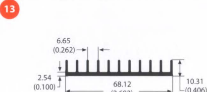
60955 0.5 lb/ft 5.87 °C/W/3in Per.=11.91
