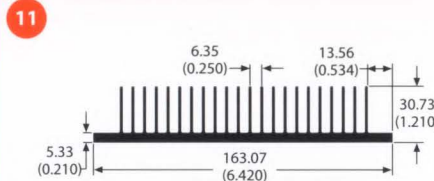
64360 3.1 lb/ft 1.24 °C/W/3in Per.=56.22
