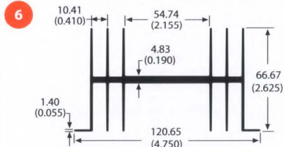
61760 1.9 lb/ft 1.81 °C/W/3in Per.=38.58
