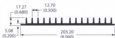
72480 2.9 lb/ft 2.33 °C/W/3in Per.=29.95
