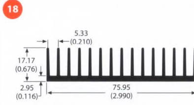
80655 1.0 lb/ft 3.12 °C/W/3in Per.=22.43
