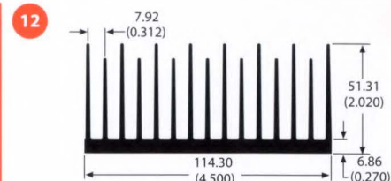
80645 3.6 lb/ft 1.23 °C/W/3in Per.=57.01
